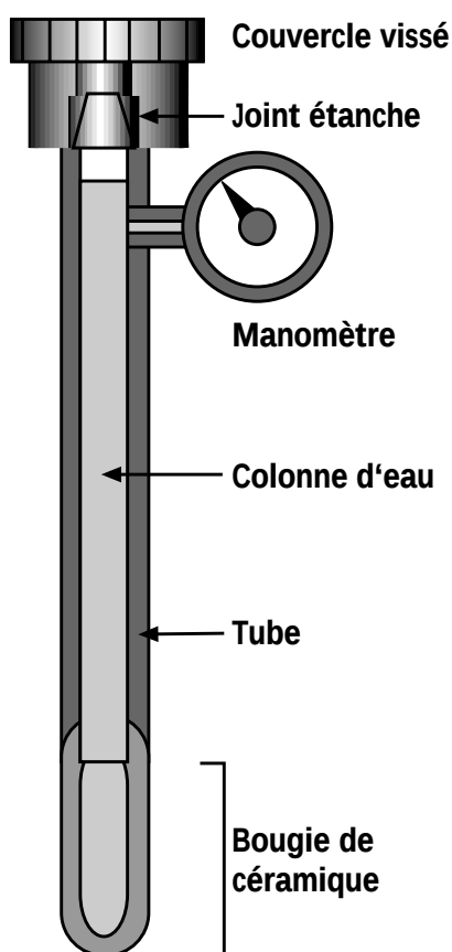
Fig. 46 : Schéma d'un tensiomètre à manomètre
